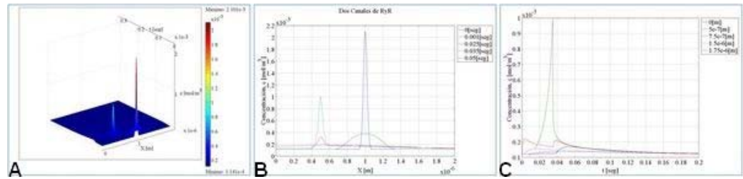
Figura 8. A. Difusión-Reacción para el disparo de un canal de RyR activado por la difusión del disparo del canal central en t = 0\text{s} . Concentración en función de la Posición y del Tiempo. B. Concentración vs Posición, en tiempos diferentes. C. Concentración vs Tiempo, en puntos diferentes del dominio
