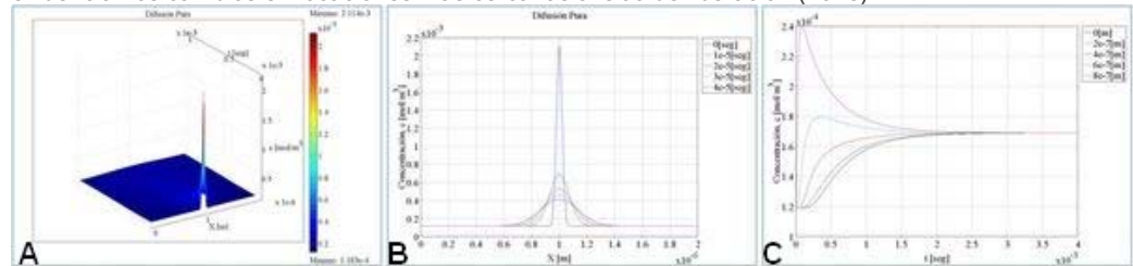
Figura 3. A: Difusión Pura para el disparo del canal central de RyR en t = 0 \text{ s} . No está presente la Calmodulina. Concentración en función de la Posición y del Tiempo. B: Concentración vs Posición, en tiempos diferentes. C: Concentración vs Tiempo, en puntos diferentes del dominio.
