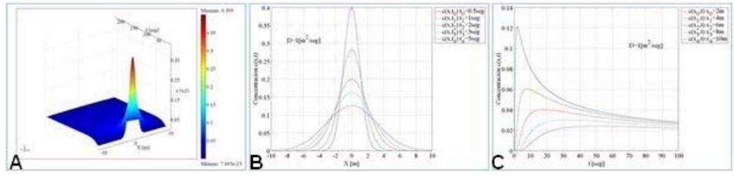
Figura 4 A. Solución analítica de la ecuación difusión pura. Concentración en función de la Posición y del Tiempo. B. Concentración Vs Posición para diferentes Tiempos. C. Concentración Vs Tiempo para diferentes puntos del dominio.
