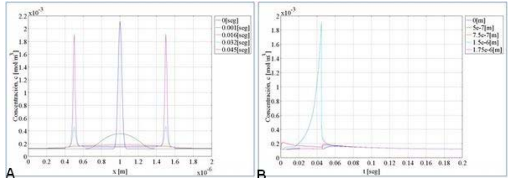
Figura 11. A. Difusión-Reacción para el disparo de tres canales de RyR. Concentración de Calmodulina de 30 μM. Concentración vs Posición, en tiempos diferentes. B. Concentración vs Tiempo, en puntos diferentes del dominio.
