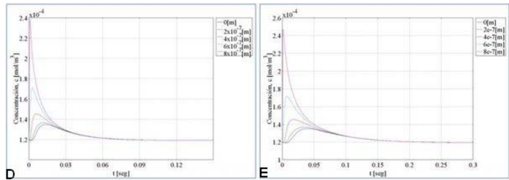
Figura 6. A. Concentración de Calmodulina 40 mM. Difusión-Reacción para el disparo del canal central de RyR y la acción de J_{serca} y J_{fuga} . Concentración en función de la Posición y del Tiempo. B. Concentración vs Posición, en tiempos diferentes. C. Concentración vs Tiempo, en puntos diferentes del dominio. D: Concentración de Calmodulina de 10 mM. Difusión-Reacción para el disparo del canal central de RyR y la acción de J_{serca} y J_{fuga} . Concentración vs Tiempo, en puntos diferentes del dominio. E: Concentración de Calmodulina de 30 \mu M Difusión-Reacción para el disparo del canal central de RyR y la acción de J_{serca} y J_{fuga} . Concentración vs Tiempo, en puntos diferentes del dominio.
