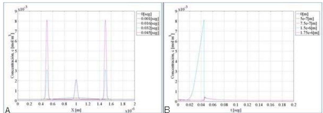
Figura 12. A. Difusión-Reacción para el disparo de tres canales de RyR; Concentración de Calmodulina 10 μM. Concentración vs Posición, en tiempos diferentes. B. Concentración vs Tiempo, en puntos diferentes del dominio.
