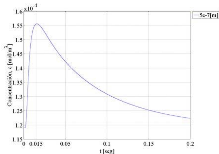
Figura 7: Concentración Vs Tiempo en x = 0.5 \mu m . Difusión del disparo en t = 0 del canal central de RyR
