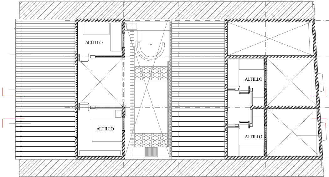
PLANTA ALTILLOS
