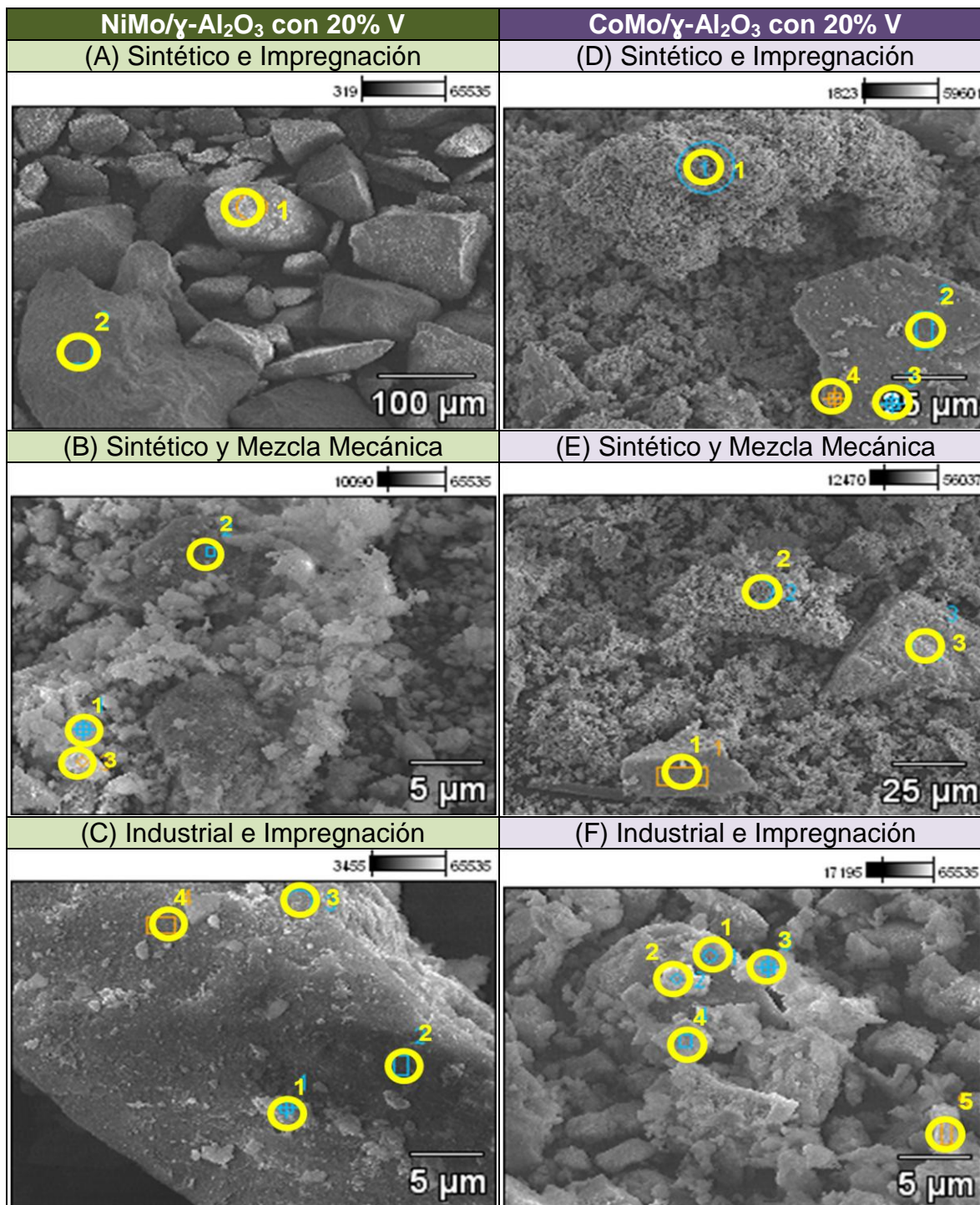
Figura 1. Microscopía Electrónica de Barrido después de la Hidrodesulfuración.
