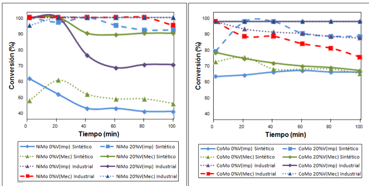
Figura 3. Conversión en HDS de los sólidos NiMo/Al 2 O 3 y CoMo/Al 2 O 3 .
