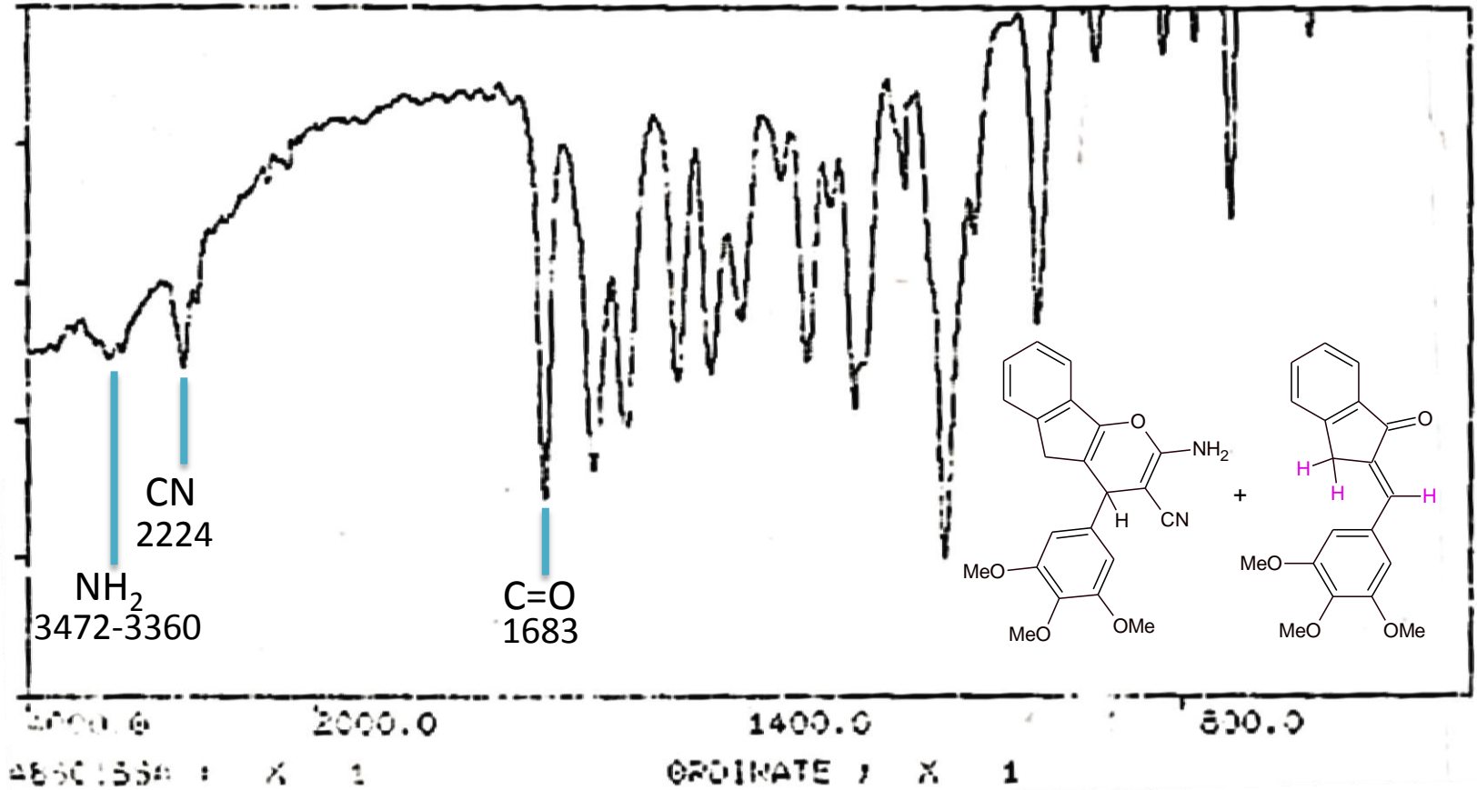
ESPECTRO IR KC6 DISCO KBR
