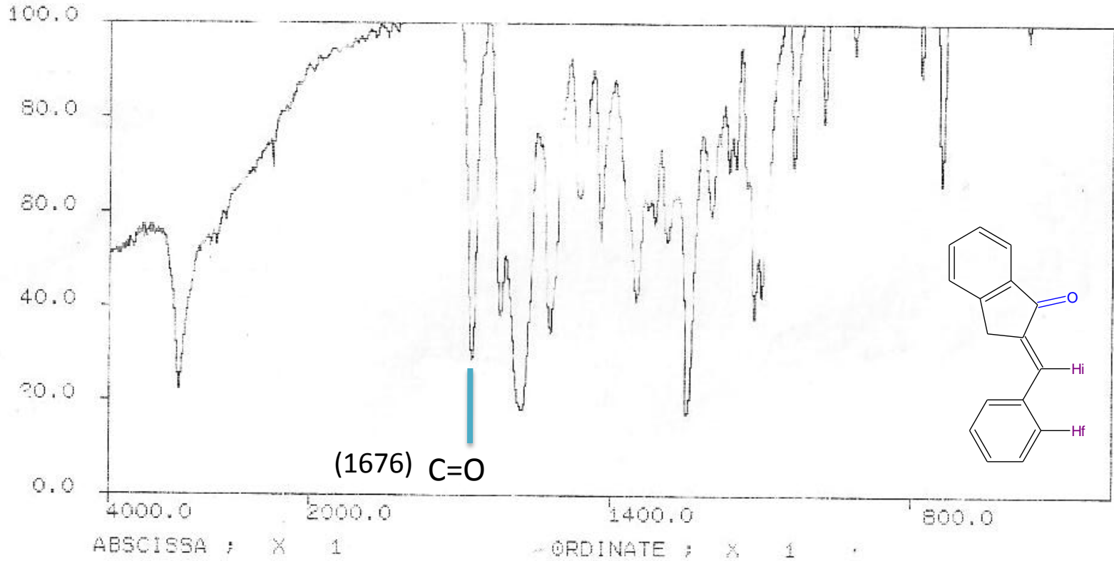
ESPECTRO IR KC-5 DISCO KBr
