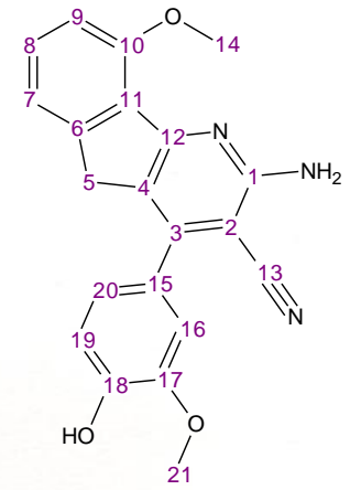
ESPECTRO RMN 13 C KC2-23 SOLVENTE: DMSO-D6 FRECUENCIA: 69MHZ
