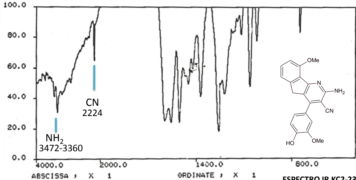
ESPECTRO IR KC2-23 DISCO KBR
