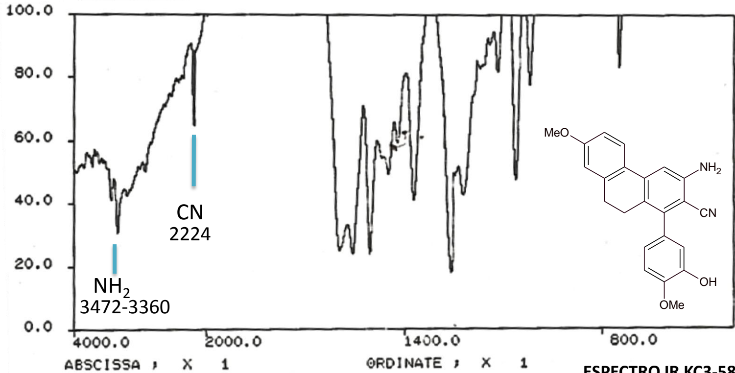
ESPECTRO IR KC3-58 DISCO KBR
