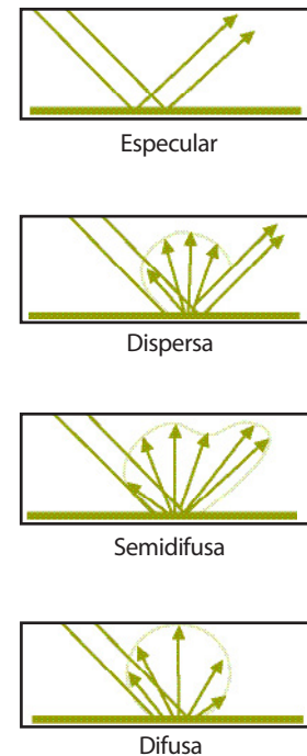
Figura 4 Tipos de reflexión de la luz en función del material y color de la superficie
