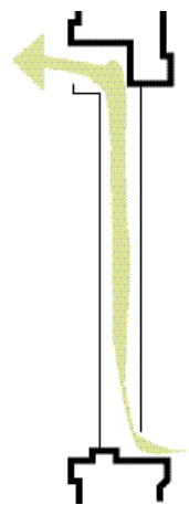
Figura 100 Detalle de ventana doble vidrio ventilada
