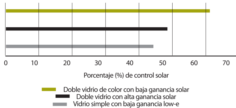
Figura 95, Gráfico 12 Comportamiento térmico de ventana de doble cristal con cámara de gas Fuente: Datos tomados de www.efficientwindows.org/glazing_double.html
