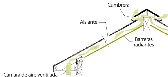
Figura 63 Integrando estrategias de diseño en los techos Fuente: Basado en Field Guide for Energy Performance, Confort and Value in Hawai Home.
