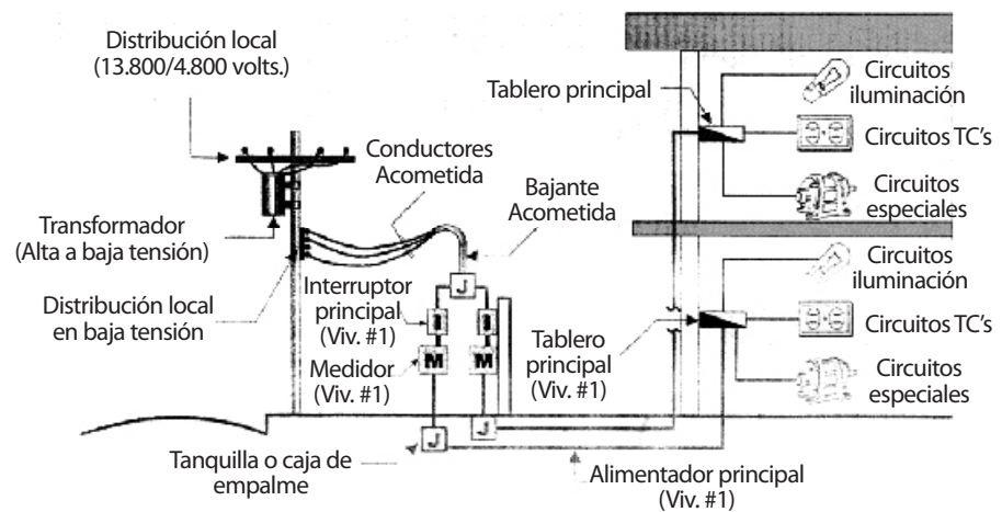
Gráfico 14 Acometida y sistema eléctrico para vivienda bifamiliar Fuente: Guías Docentes del Profesor Juan Cámara UC.V.
