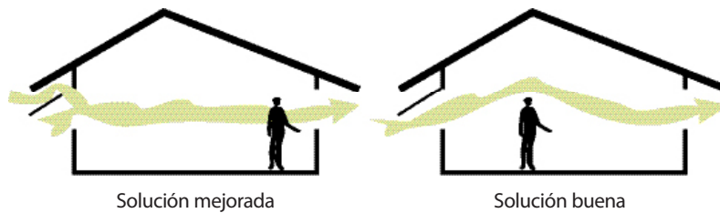
Figura 38 Uso de parasoles para dirigir la ventilación natural en el interior de los espacios
