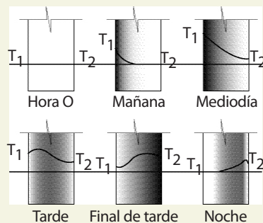
Figura 54 Mecanismo de inercia térmica en una pared Fuente: Basado en Santimouris et al. Passive cooling of Building. James & James (1996).
