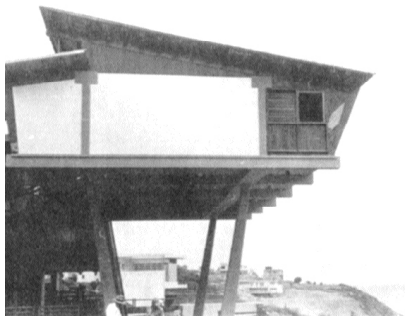
Figura 28 Vivienda elevada del suelo para estimular la circulación del aire alrededor y dentro de los ambientes
