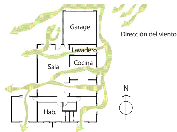
Figura 31 Diseño inadecuado para la ventilación cruzada Fuente: Basado en Field Guide for Energy Performance, Comfort and Value in Hawaii Home.
