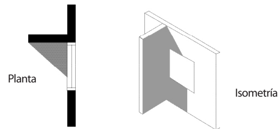
Figura 89 Detalle de planta e isometría de protector solar vertical para bloquear ángulos bajos del sol en fachadas este y oeste
