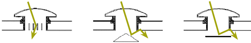
Figura 68 Opciones de cúpulas cenitales con difusores y espejos
