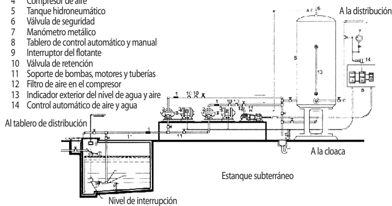
Figura 120 Sistema de bombeo de aguas blancas
