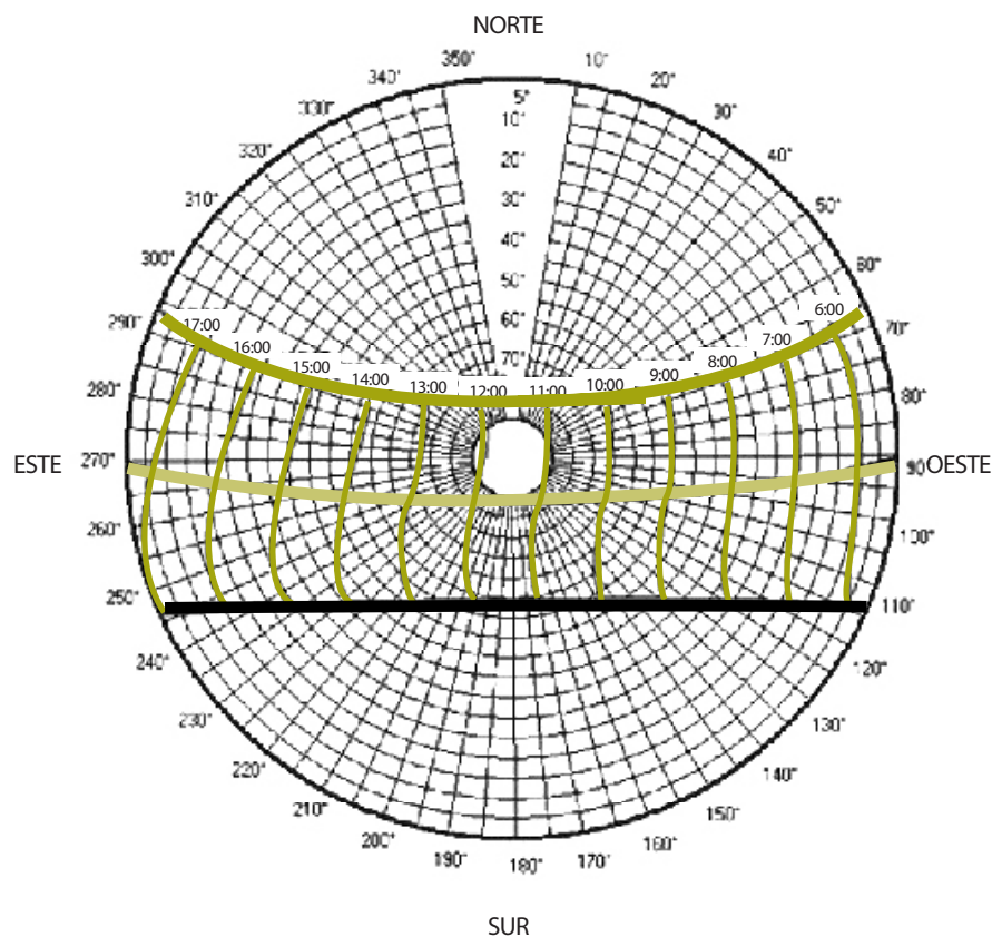
Figura 87 Localización: Caracas • Latitud: 10,6° N • Longitud: 67,0° Este • Hora: 2:00 pm Junio 21 • Marzo 21 • Septiembre 21 • Enero 1 • Diciembre 31 • Diciembre 21 Fuente: Elaboración propia en base al software Programa IES, Sunpath.
