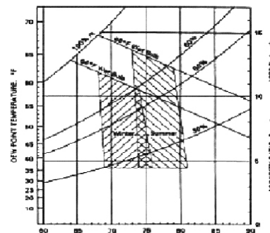
Gráfico 17 Zona de confort en verano e invierno según ASHRAE Fuente: Siem Et al. Guía de Operaciones de Ahorro de Energía Eléctrica en Edificaciones Públicas. MEM - 2002.
