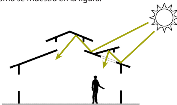
Figura 66 Aprovechamiento de la iluminación natural a través de aberturas en techo
