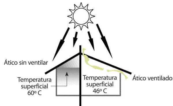
Figura 58 Comparación de los efectos de áticos ventilados y no ventilados en la temperatura del aire de los espacios interior
