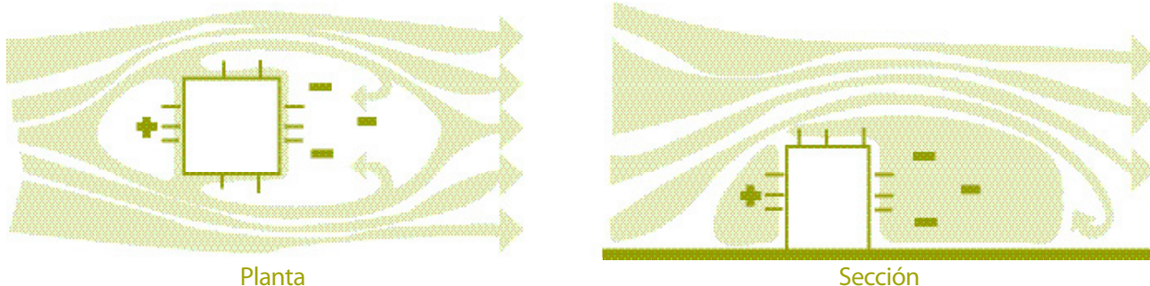
Figura 2 Campos de presión y comportamiento del aire alrededor de la edificación
