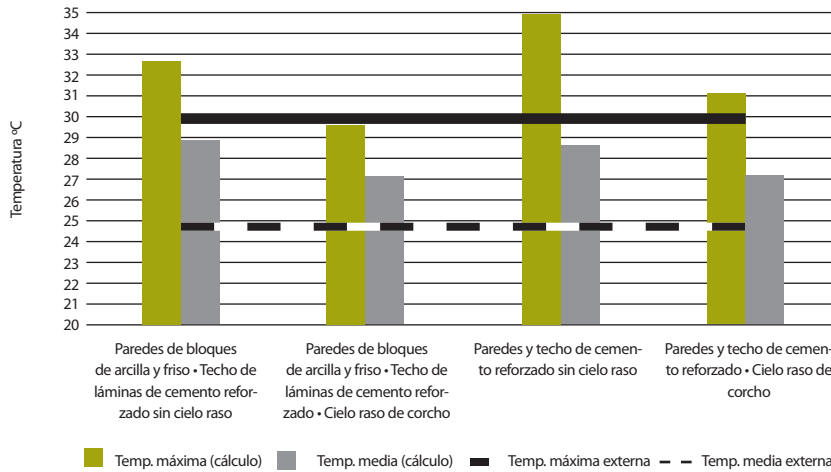
Gráfico 9 Valores de temperatura obtenidos analíticamente para diferentes sistemas constructivos sin y con material aislante Fuente: Datos tomados de Hobaica-Sosa-Rosales «Influencia de las características térmicas de los componentes constructivos en la temperatura del aire interior de viviendas», Revista Interciencia.
