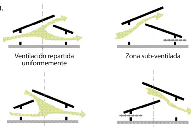
Figura 65 Influencia de la ubicación de las aberturas en techos Fuente: Basado en CSTB. Guide sur la climatisation naturelle de l'habitat en climat Tropical-Humide.
