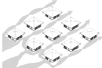
Figura 18 Ventilación pobre en una disposición lineal de las edificaciones, con caras paralelas a la dirección del viento
