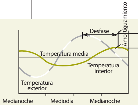
Gráfico 6 Mecanismo de inercia térmica
