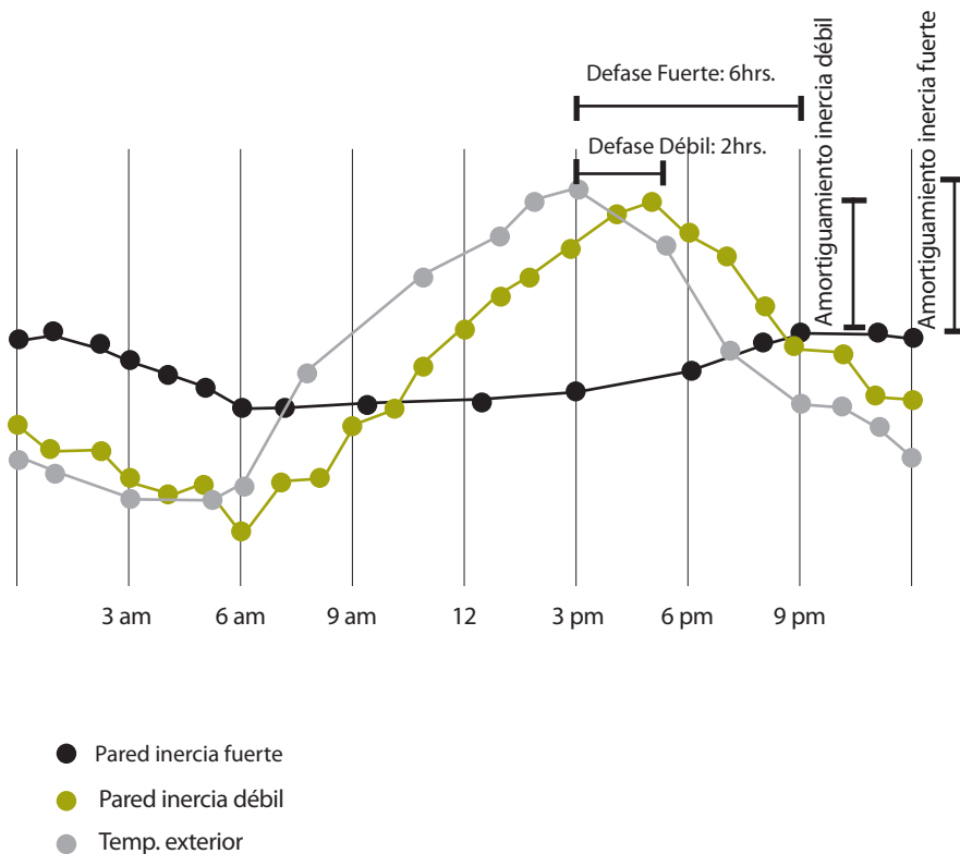
Gráfico 10 Esquema del mecanismo de inercia en paredes
