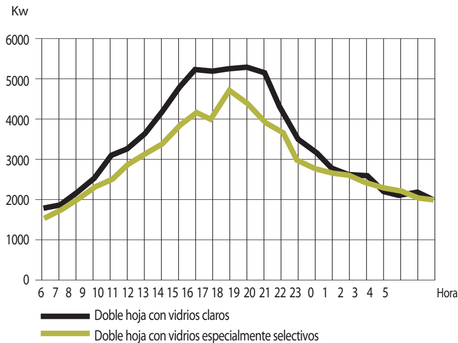
Gráfico 16 Requerimientos de potencia total del sistema de aire acondicionado con vidrios dobles claros y espectralmente selectivos
