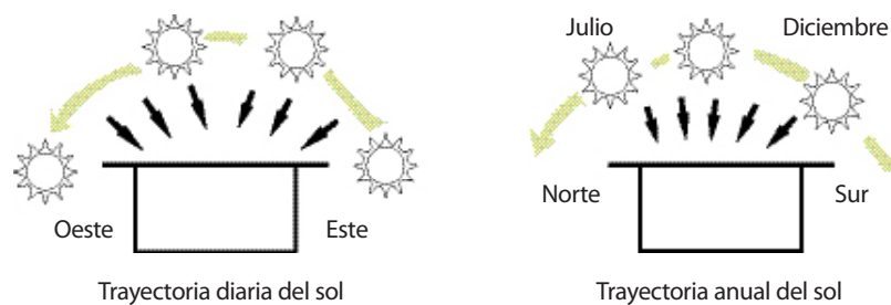
Figura 48 Incidencia solar sobre un techo plano en el trópico, latitud norte
