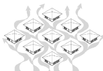
Figura 19 Buena ventilación en una disposición lineal de las edificaciones, con caras oblicuas a la dirección del viento
