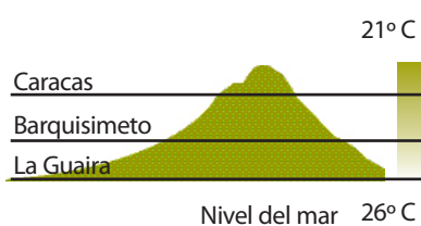
Gráfico 4 Variación de la temperatura en función de la altitud
