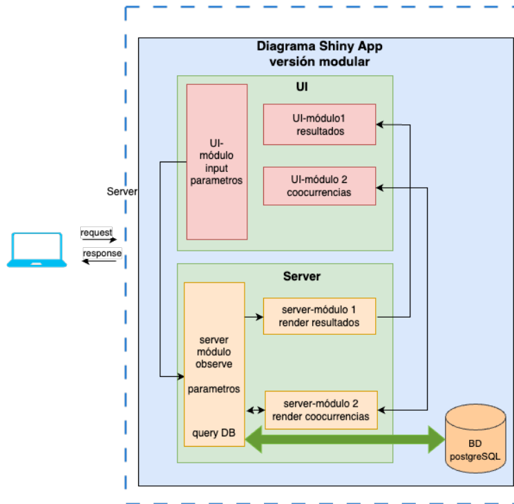
Figura 5.39: Diagrama aplicación web Shiny versión modular
