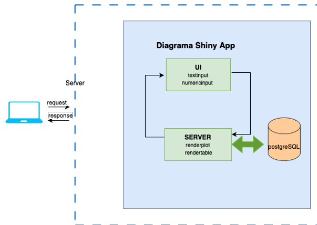
Figura 5.20: Esquema general de prototipo de la aplicación
